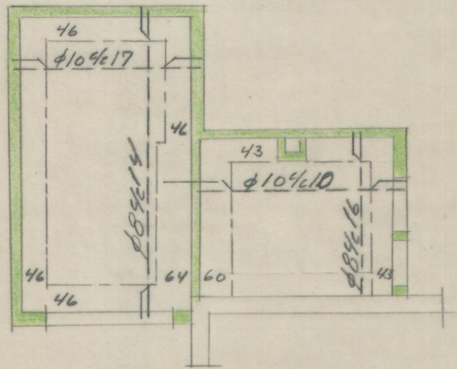
Plata 1:20
