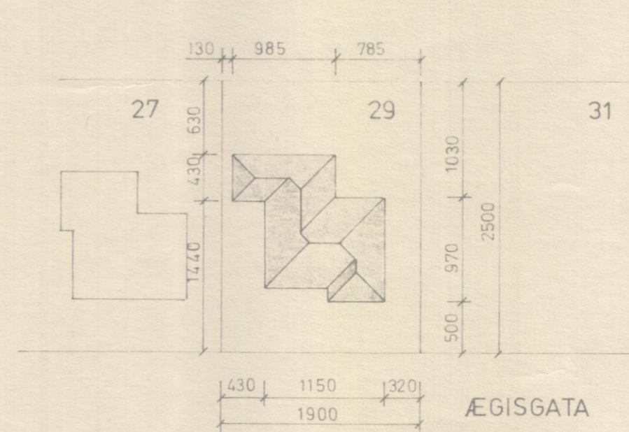
Afstöðumynd, 1:500
