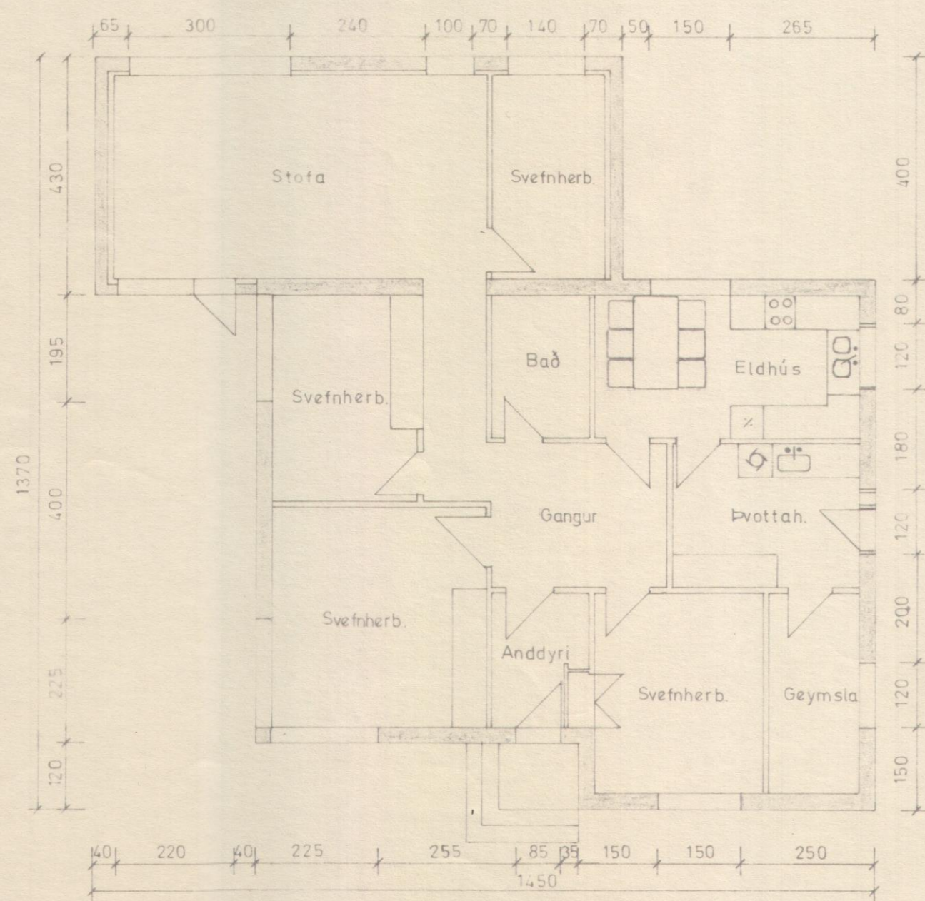
Grunnmynd, 1:100
