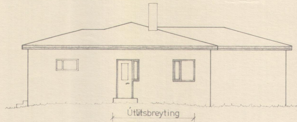
Norðurhlið, 1:100
