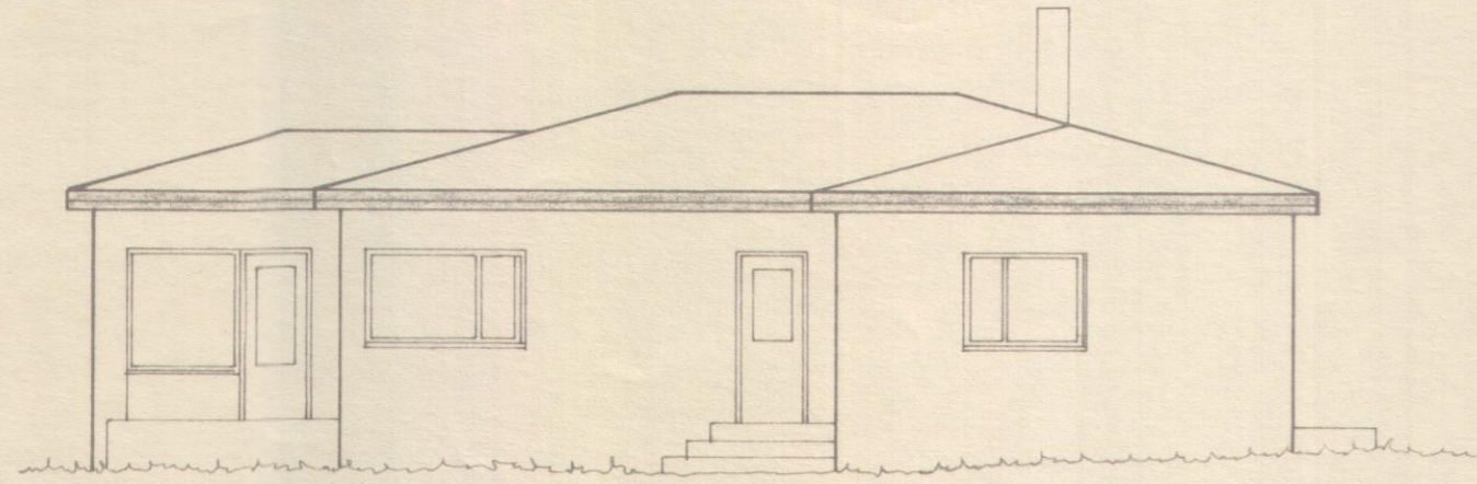
Austurhlið, 1:100
