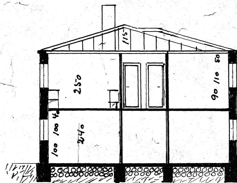
Skurðmynd ff.-ff.
