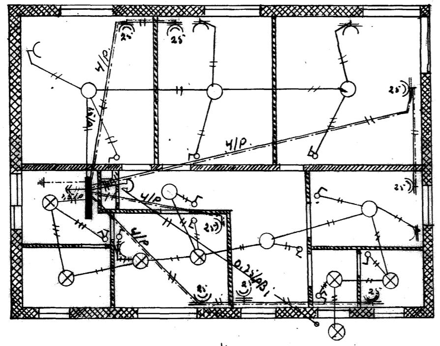
Hæð.
