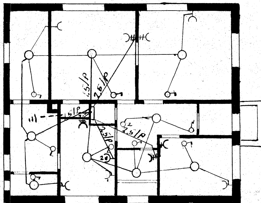
HÆÐ
