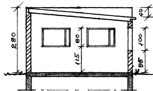
SKURDUR A-A
