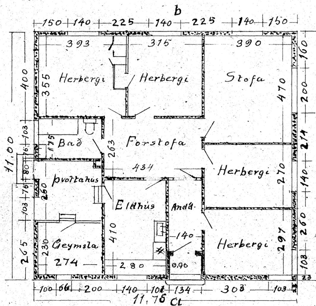
Grunnmynd
