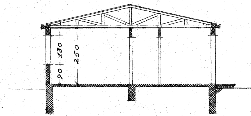
Þversniðing
