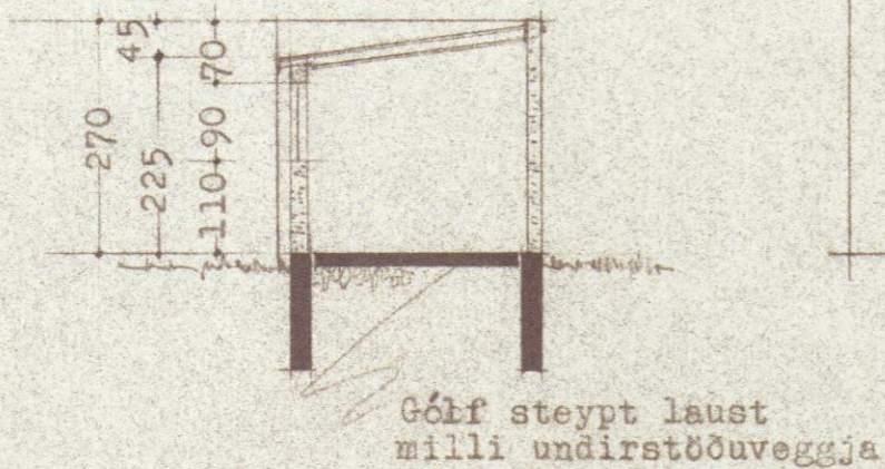
Skurður a - a
