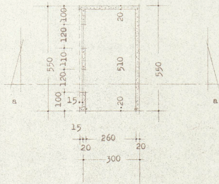
Grunnmynd bifreiðageymslu
