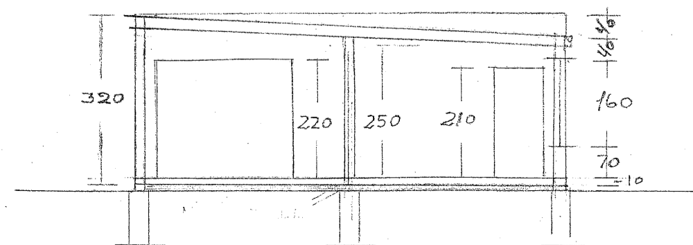
SKURÐUR A-A
