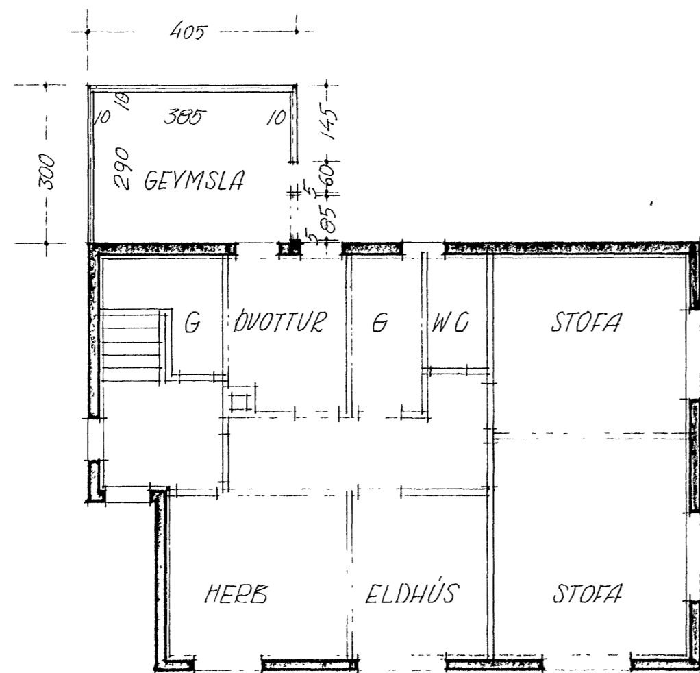
1 HÆÐ
