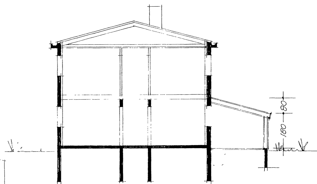
SKURÐUR
