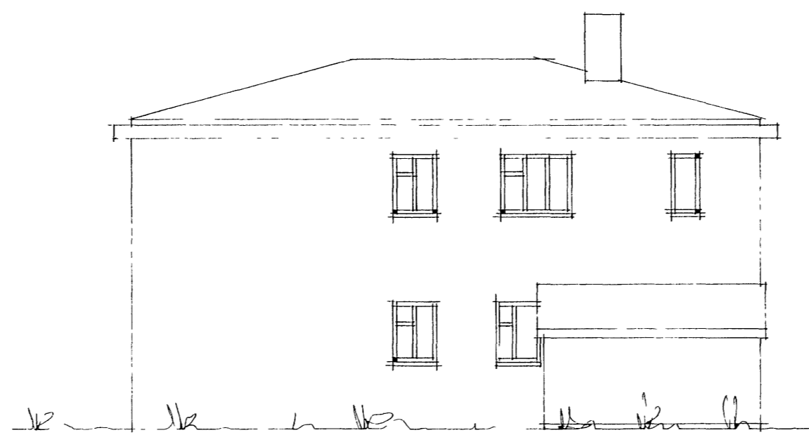
AUSTUR
