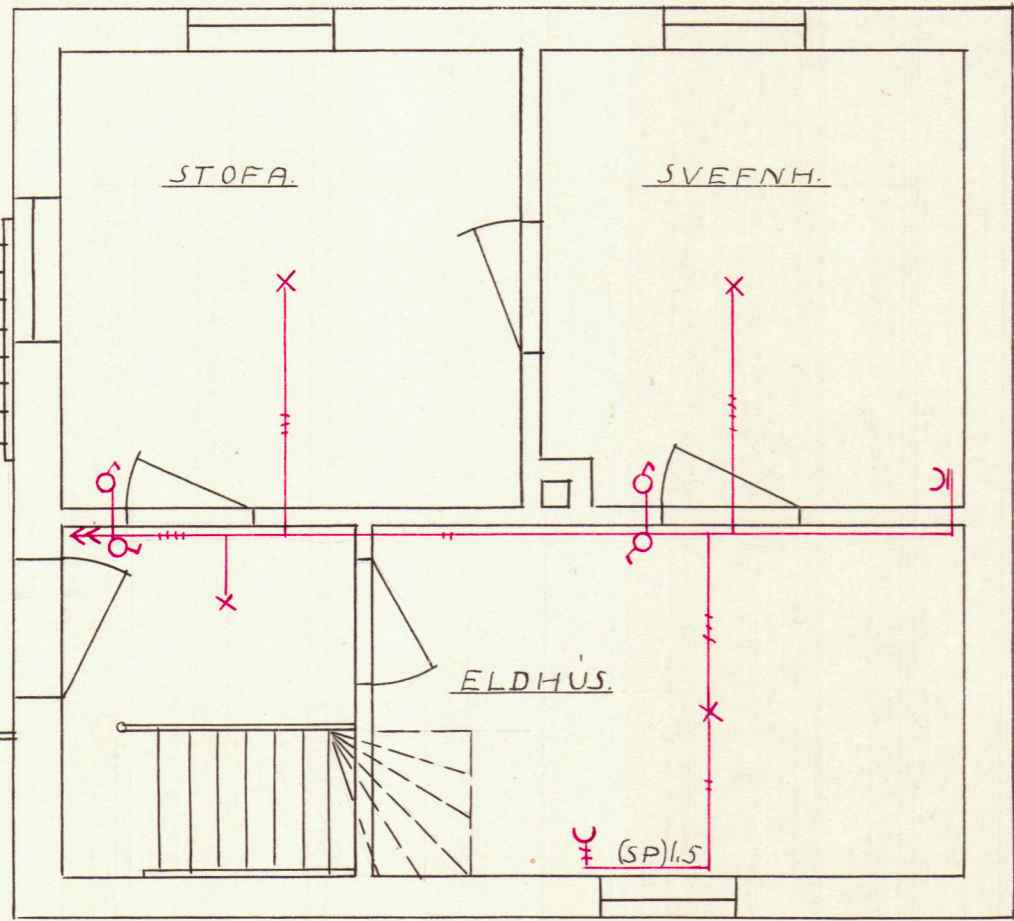
1. HÆÐ.
