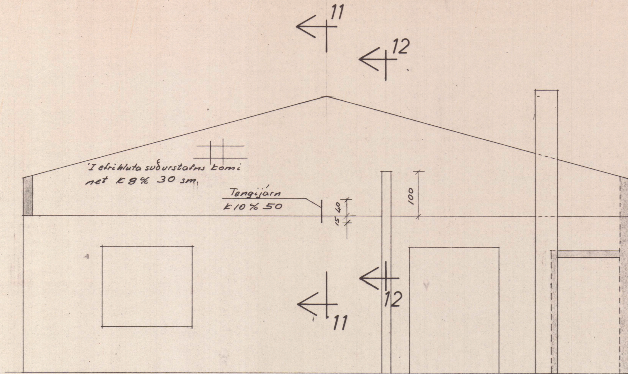
SUÐURSTAFN M:1:50
