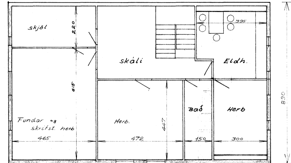
2. HÆÐ-RIS
