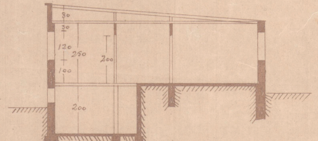
Skurður a-a.
