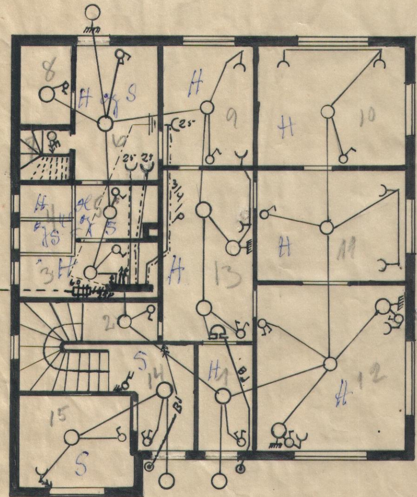
Nedri hæð
