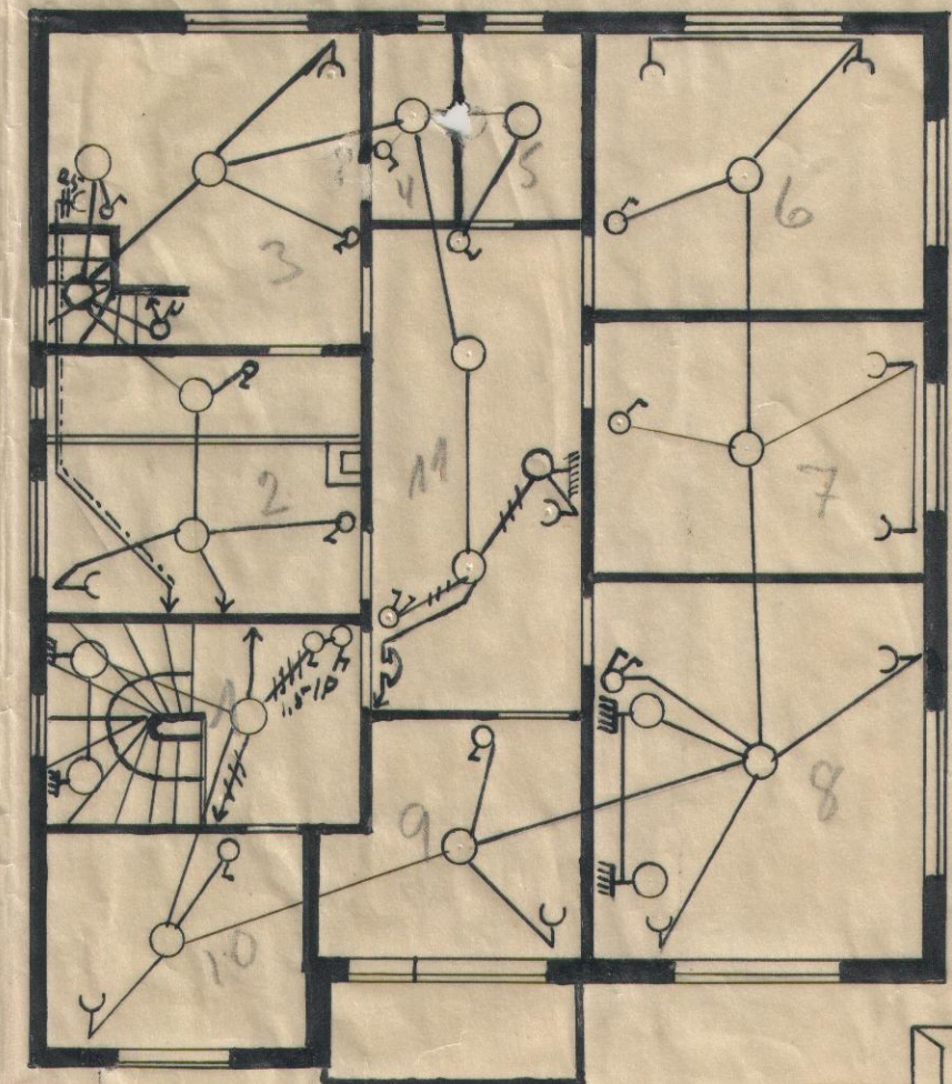
Efri hæð
