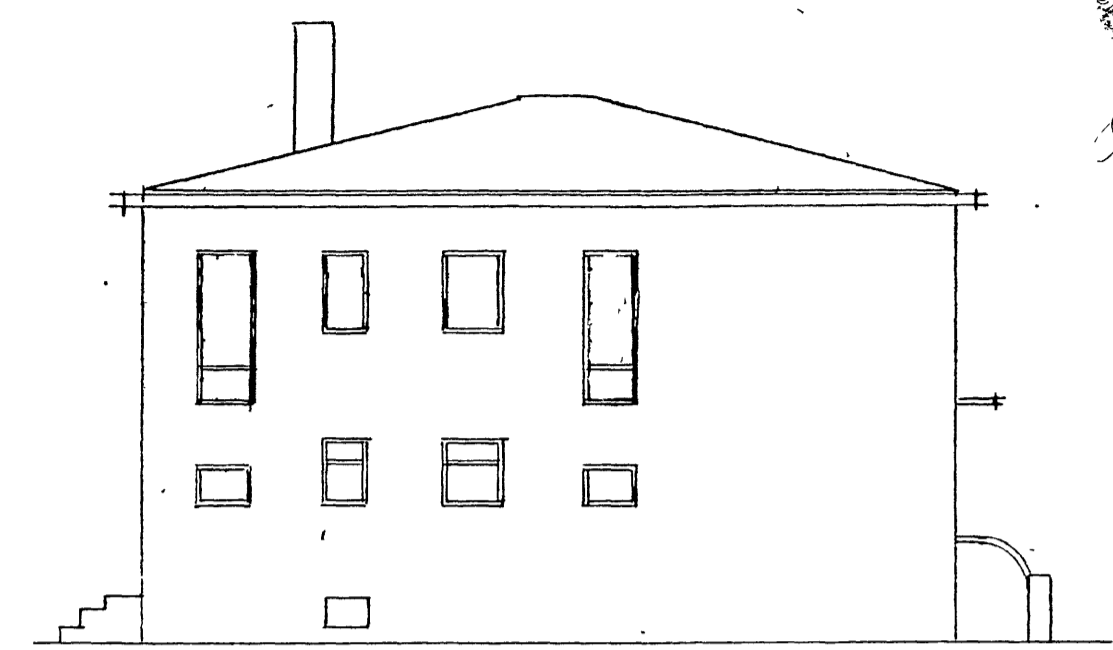
Norður.
