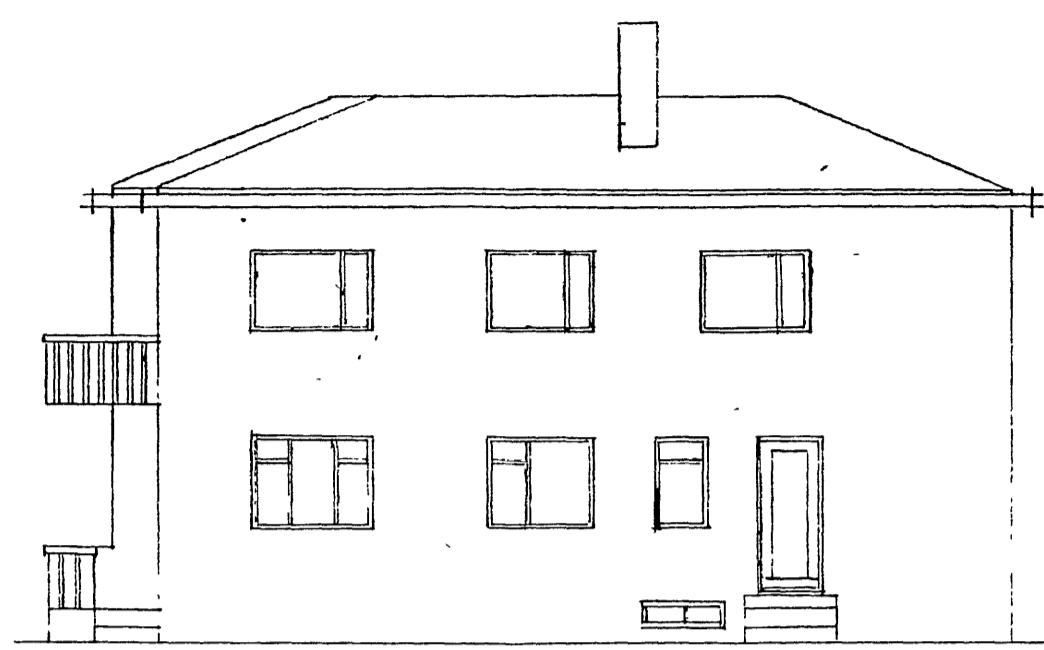
Austur.
