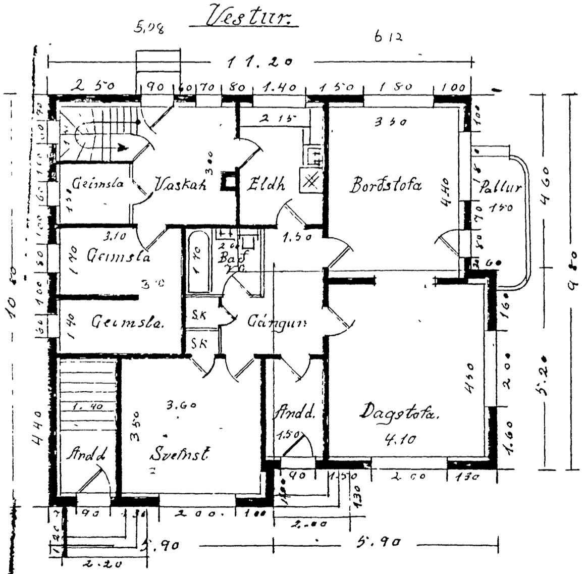
1. Hæð.
