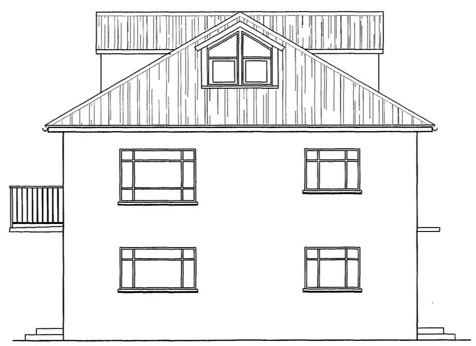
ÚTLIT SUÐUR 1:100
