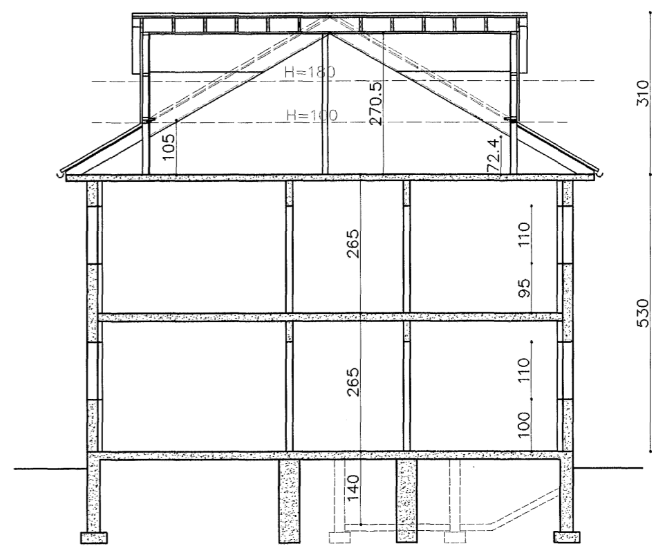
SNÍÐ A-A 1:100
