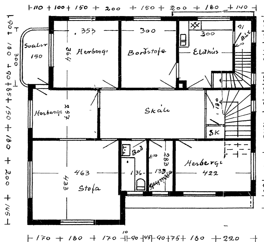
Efri hæð
