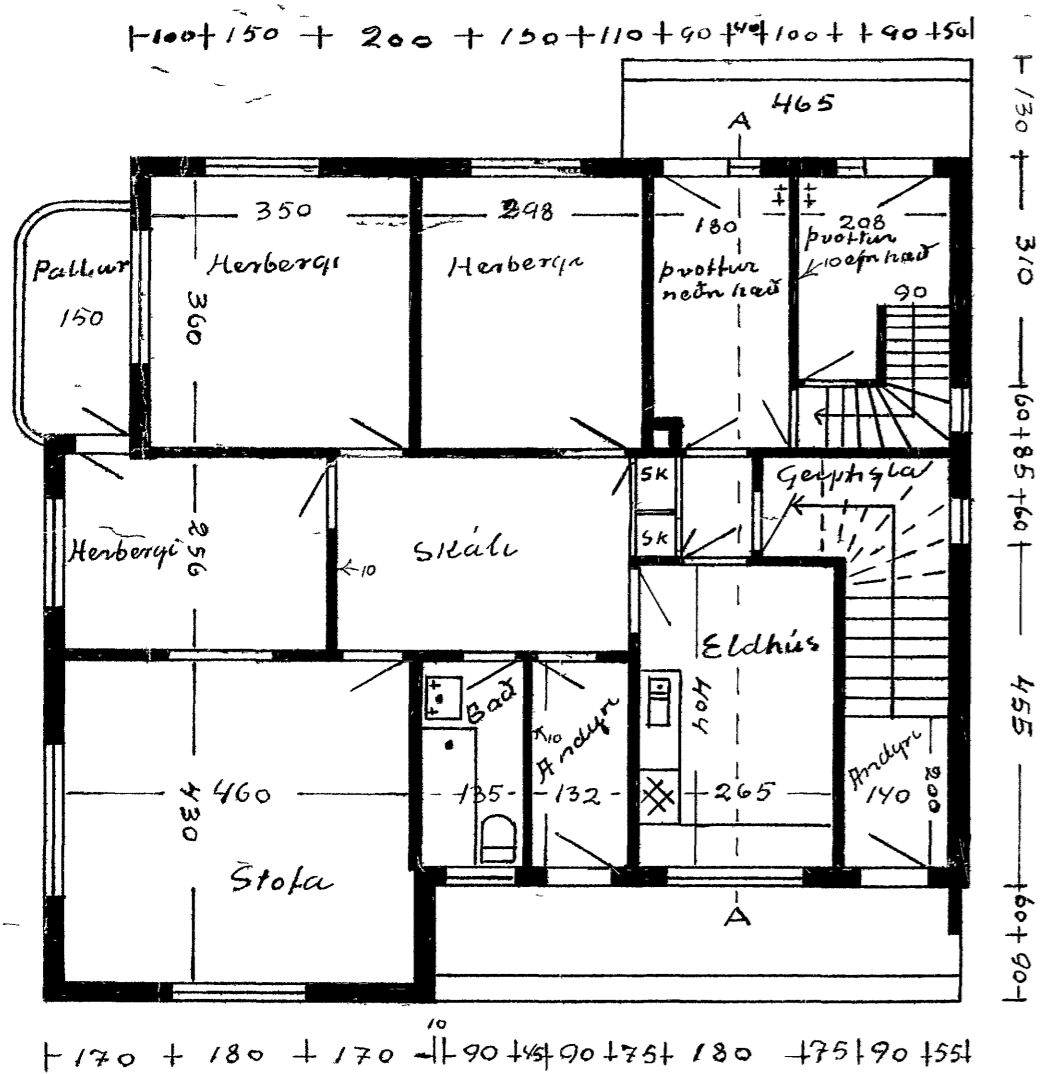
Neðri hæð
