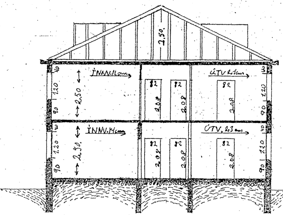
Skurður. AA
